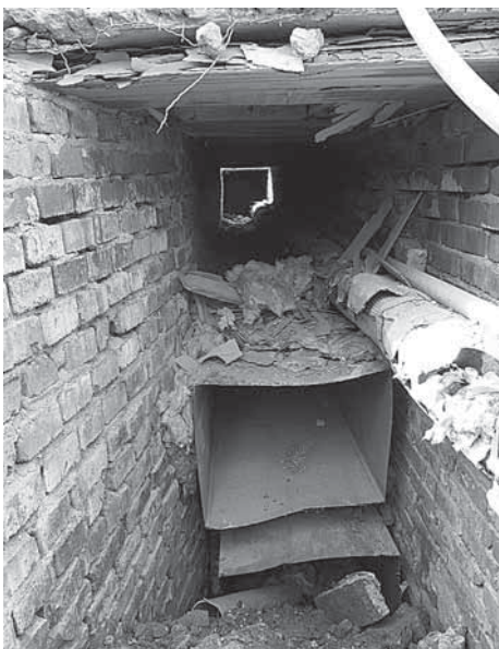
Šachta, kterou byl doposud přiváděn ohřátý vzduch z fary do kostela.
